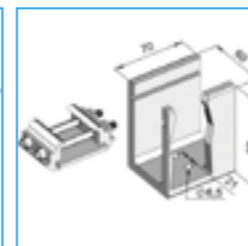
Schienenhalter Tuchstütze feststehend
