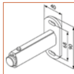
Distanzkonsole auf Fassade
