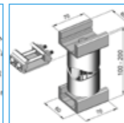
Distanzierung
