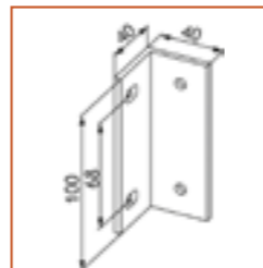
Laibungswinkel
