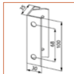
Montagewinkel auf Blendrahmen
